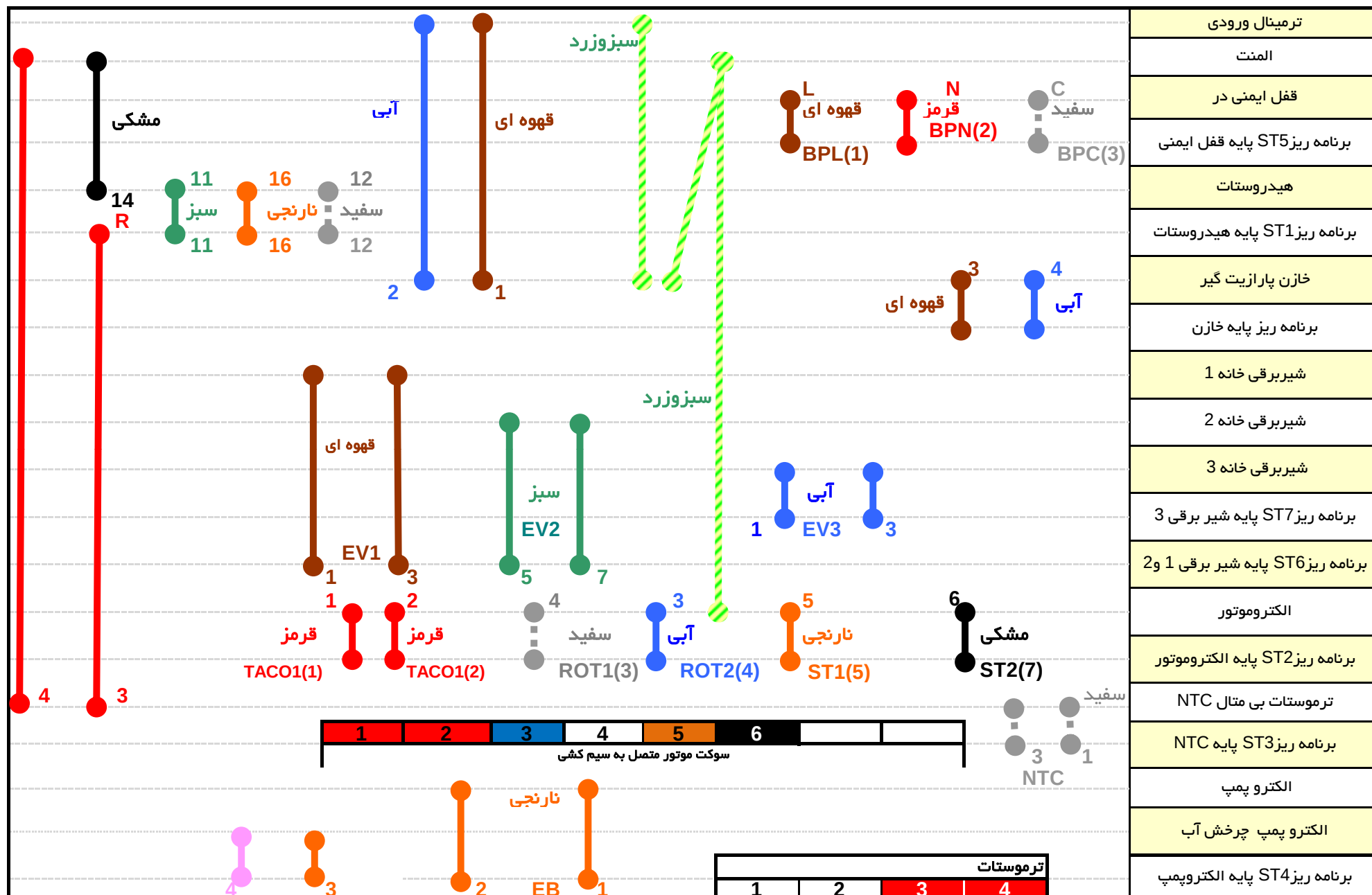
نقشه سیم کشی ماشین لباسشویی AFS-12073
